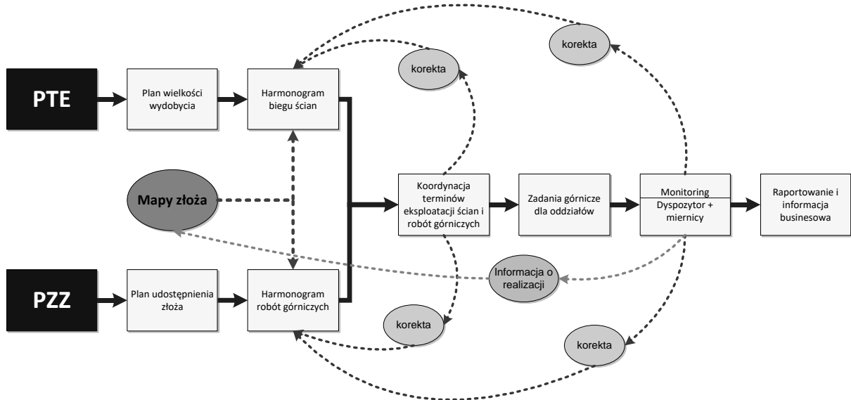
Rys 2. Proces planowania oraz monitorowania robót górniczych w kopalni węgla kamiennego
